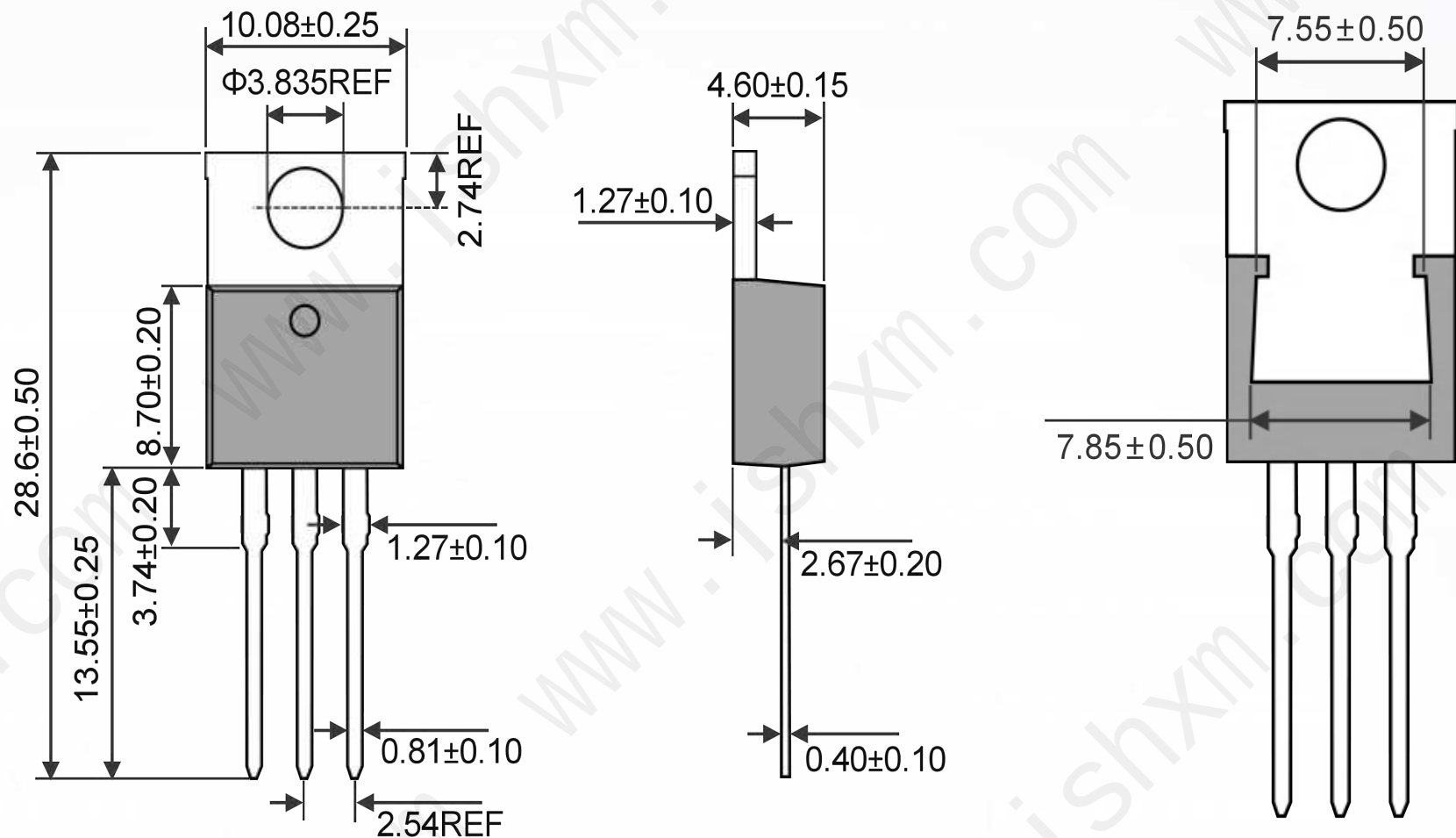
TO-220AB Unit:mm
