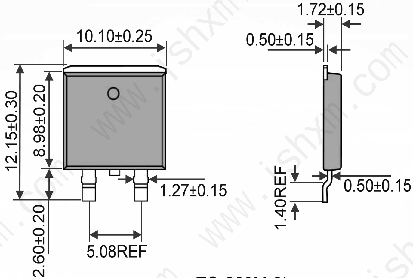
TO-263M-2L Unit:mm
