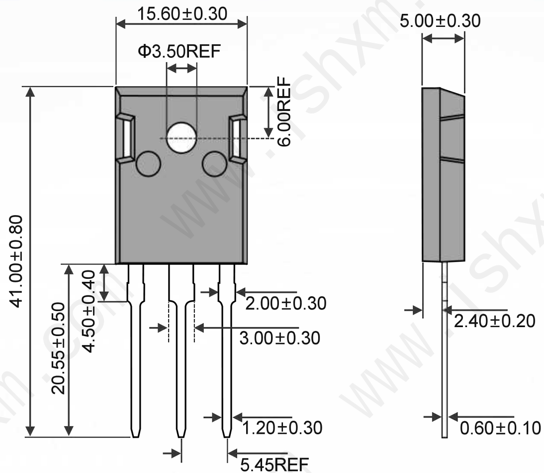
TO-247AB Unit:mm
