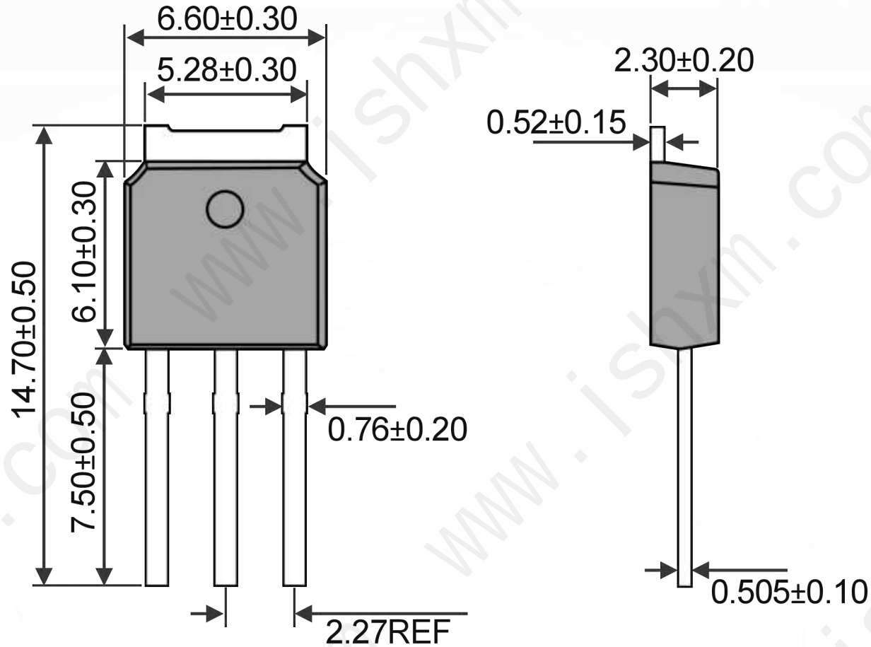
TO-251-3L Unit:mm
