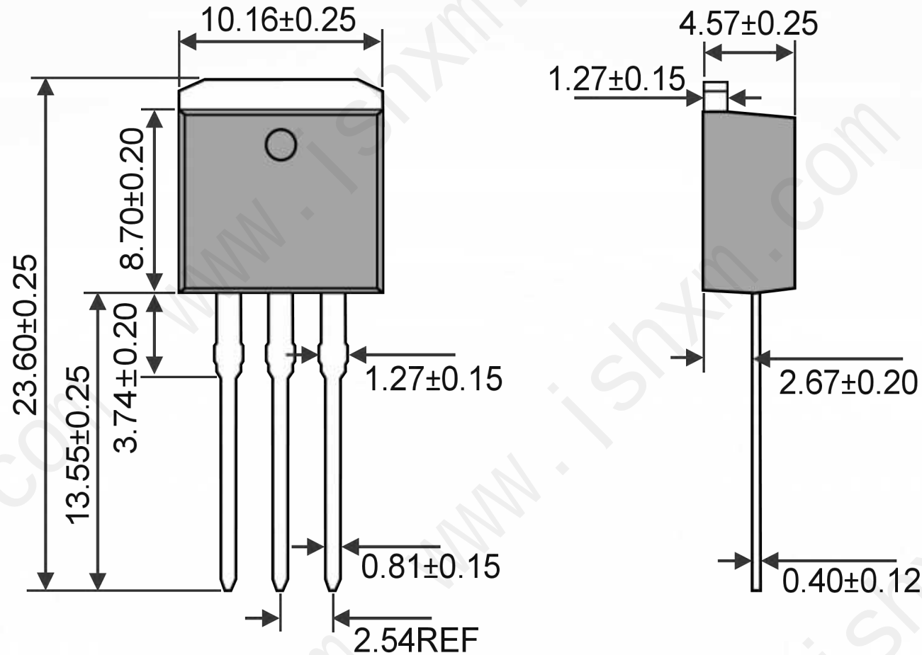
TO-262-3L-D Unit:mm
