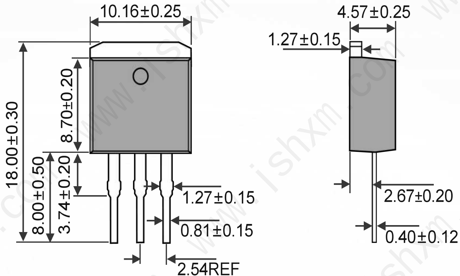
TO-262-3L Unit:mm
