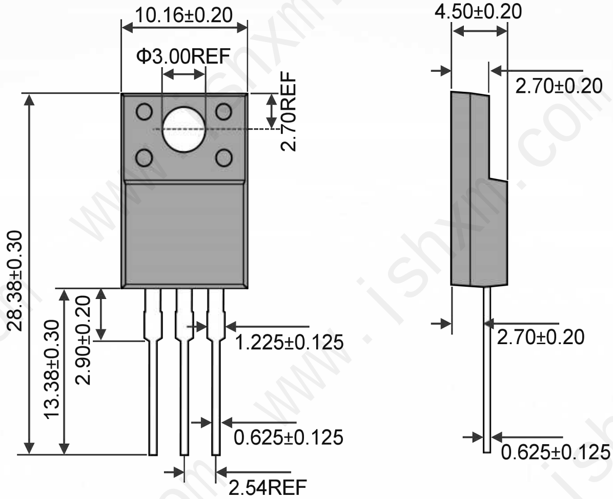
ITO-220AB Unit:mm
