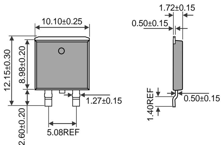
TO-263M-2L Unit:mm
