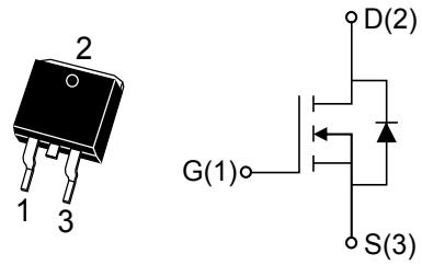
TO-263-2L
