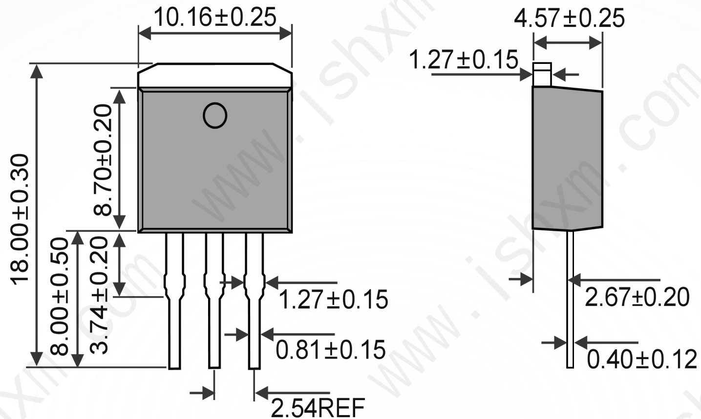
TO-262-3L Unit:mm
