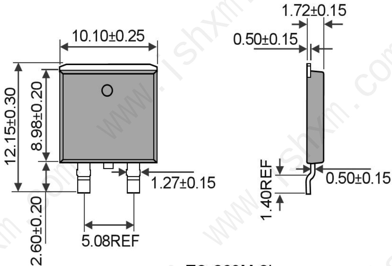
TO-263M-2L Unit:mm
