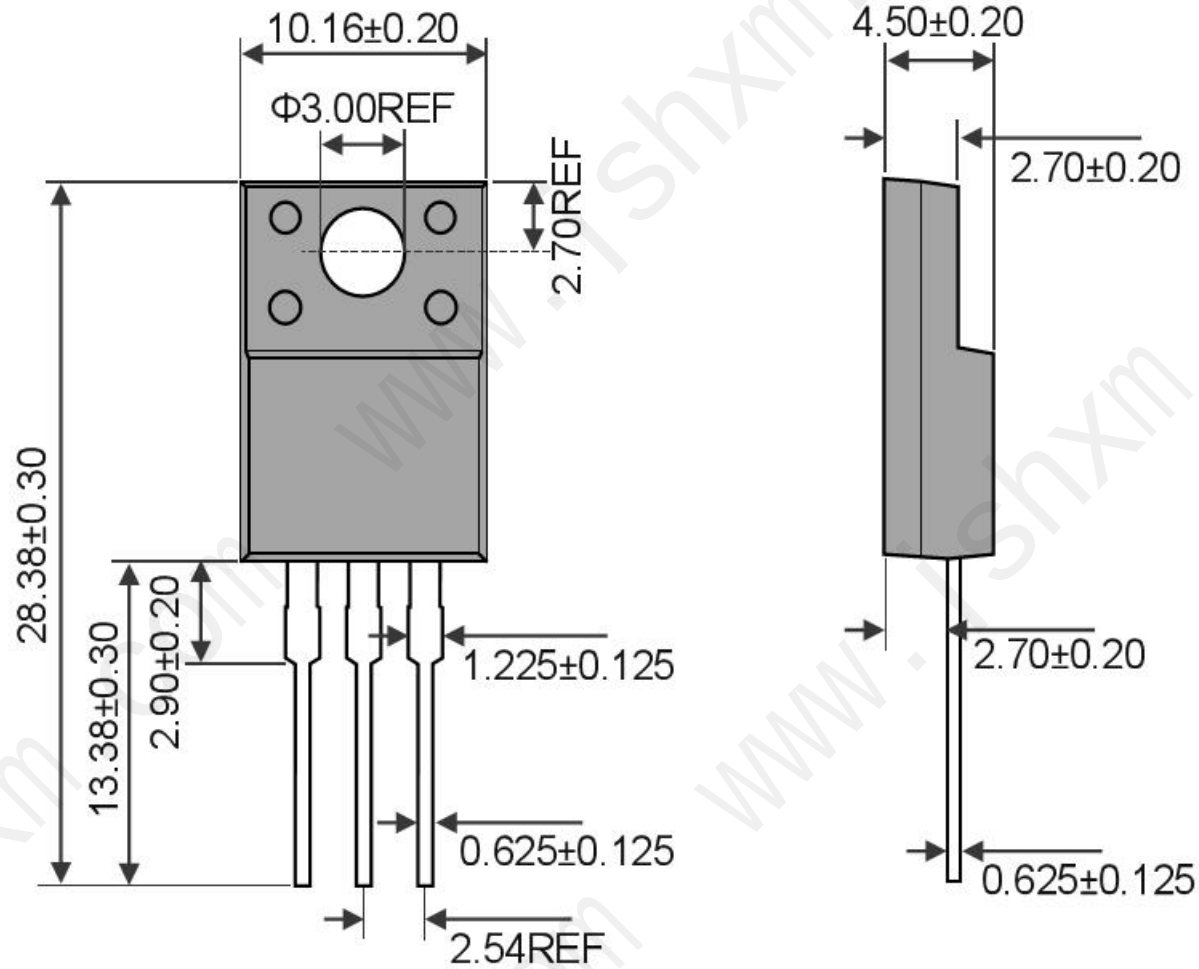
ITO-220AB Unit:mm
