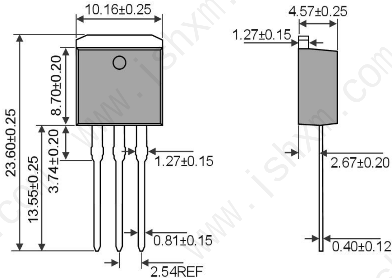
TO-262-3L-D Unit:mm
