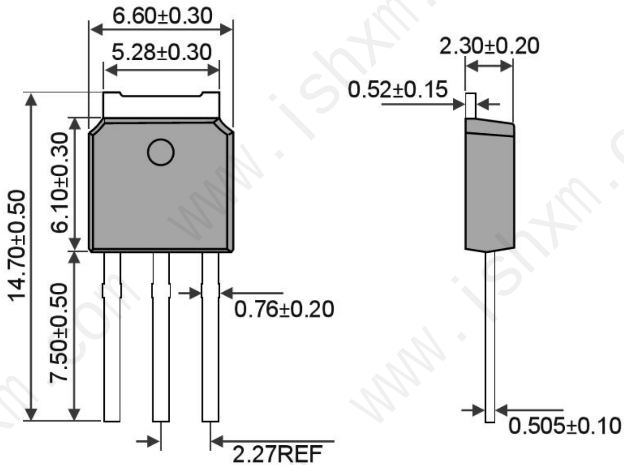
TO-251-3L Unit:mm
