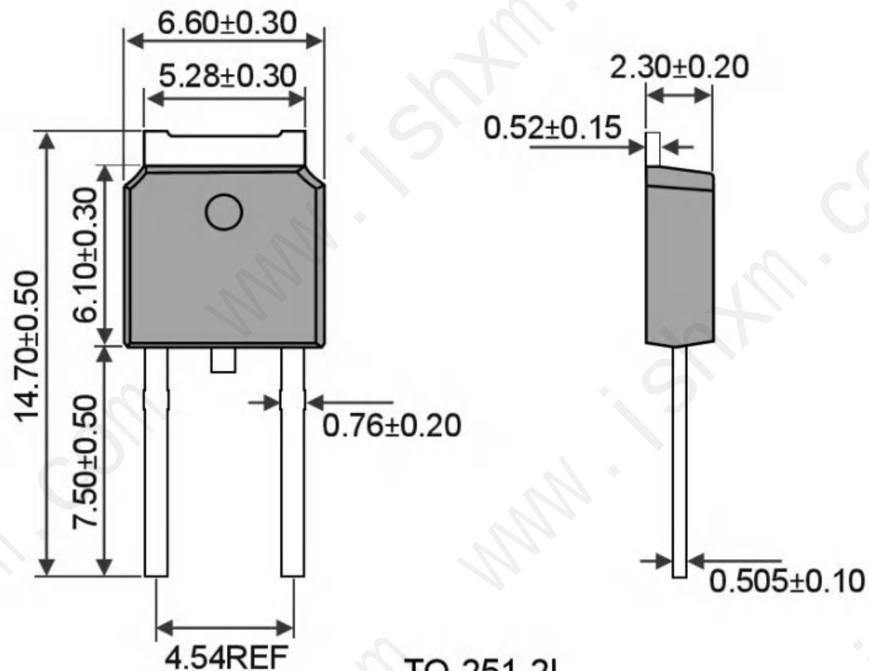
TO-251-2L Unit:mm
