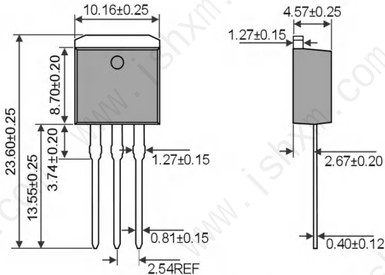
TO-262-3L-D Unit:mm
