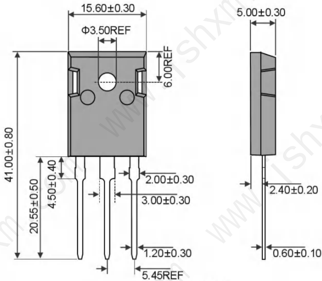
TO-247AB Unit:mm
