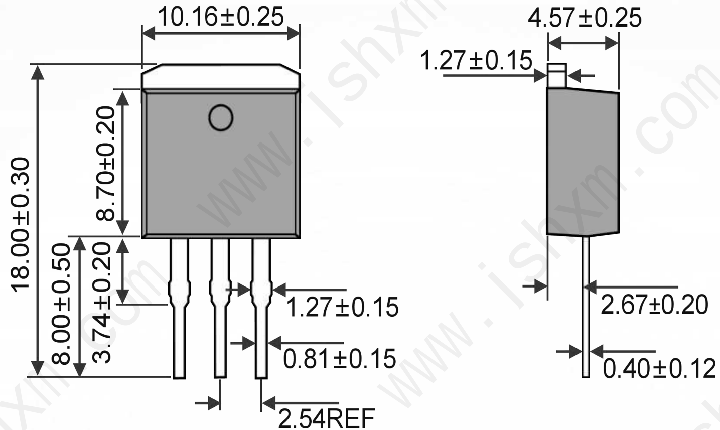
TO-262-3L Unit:mm
