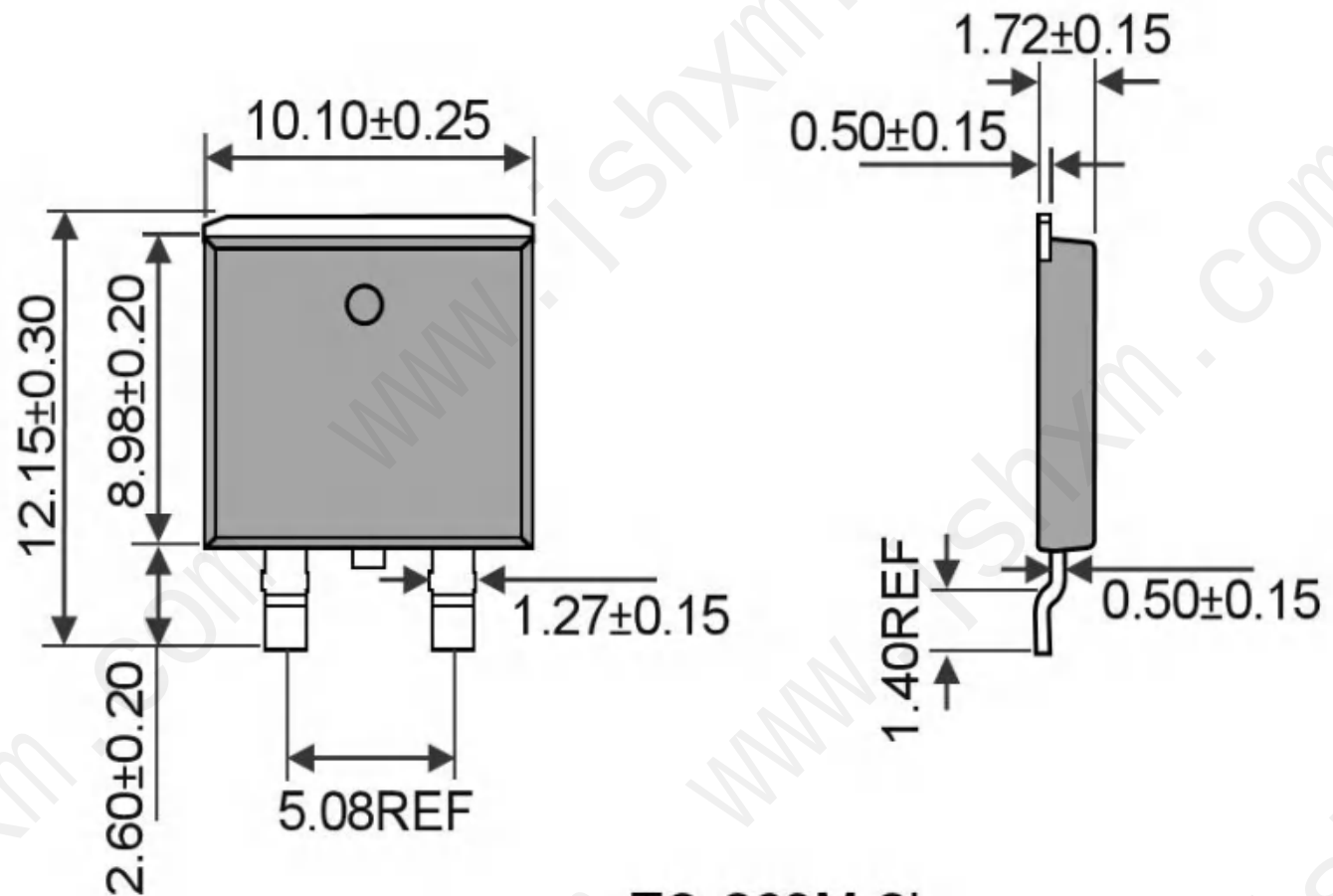
TO-263M-2L Unit:mm
