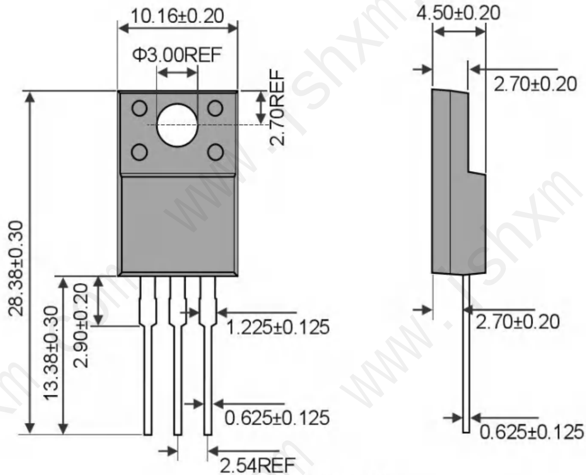
ITO-220AB Unit:mm
