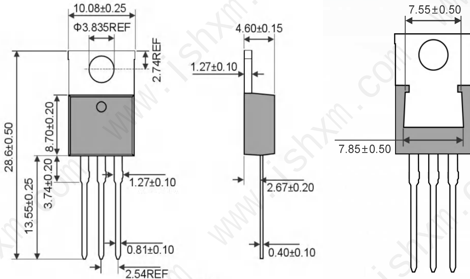
TO-220AB Unit:mm
