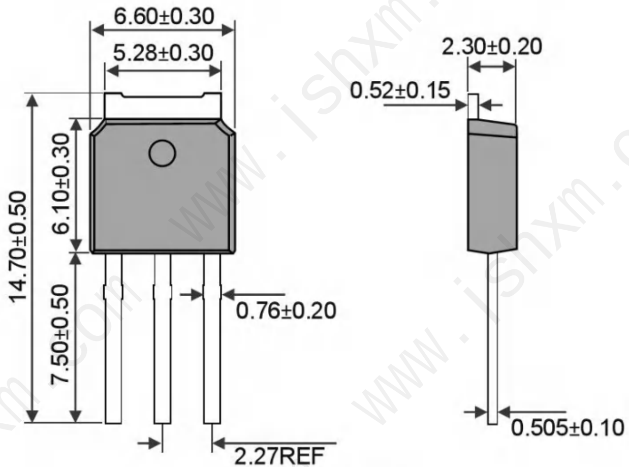
TO-251-3L Unit:mm
